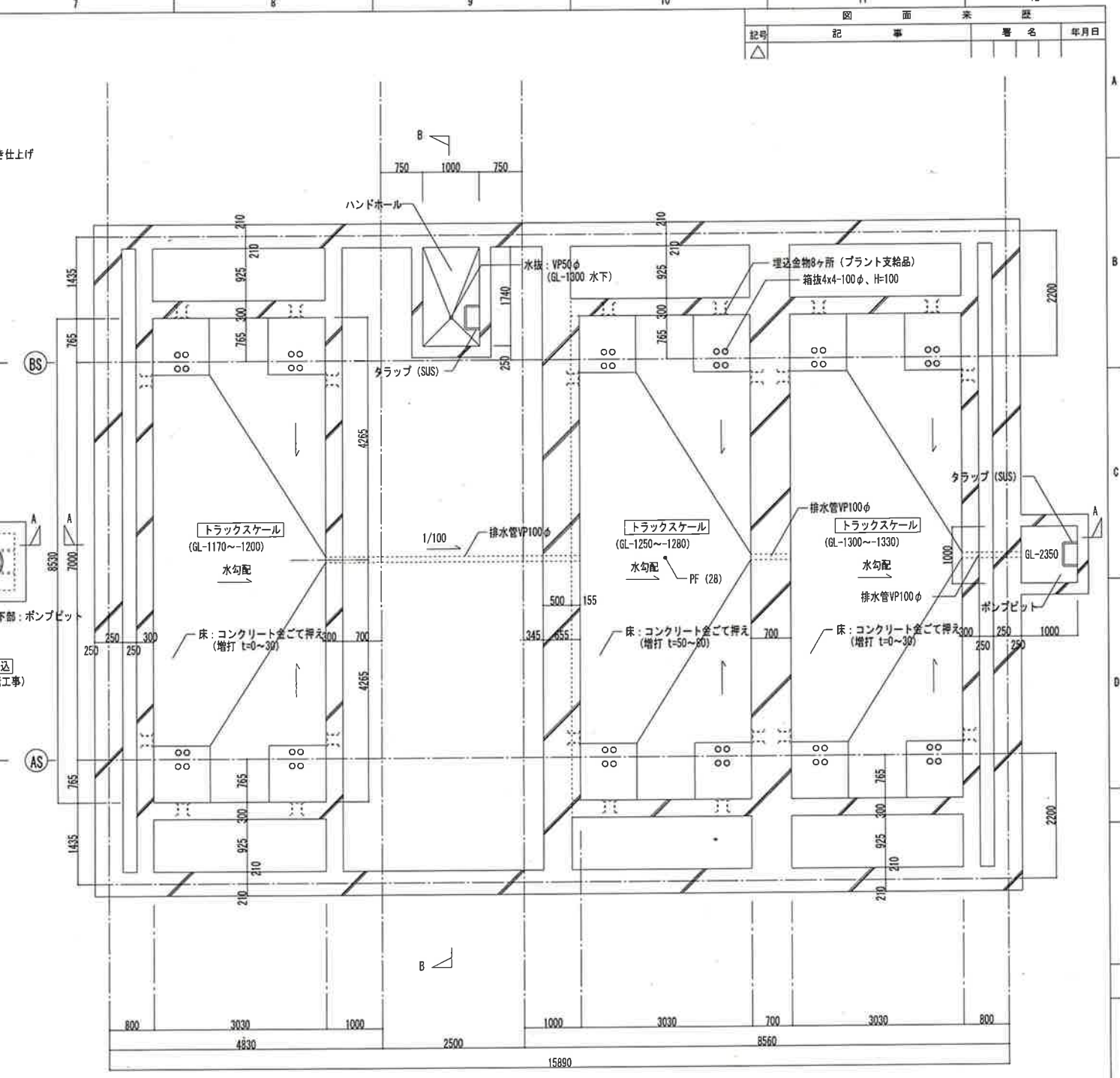
トラックスケール平面詳細図 1:50 (GL-1200)
