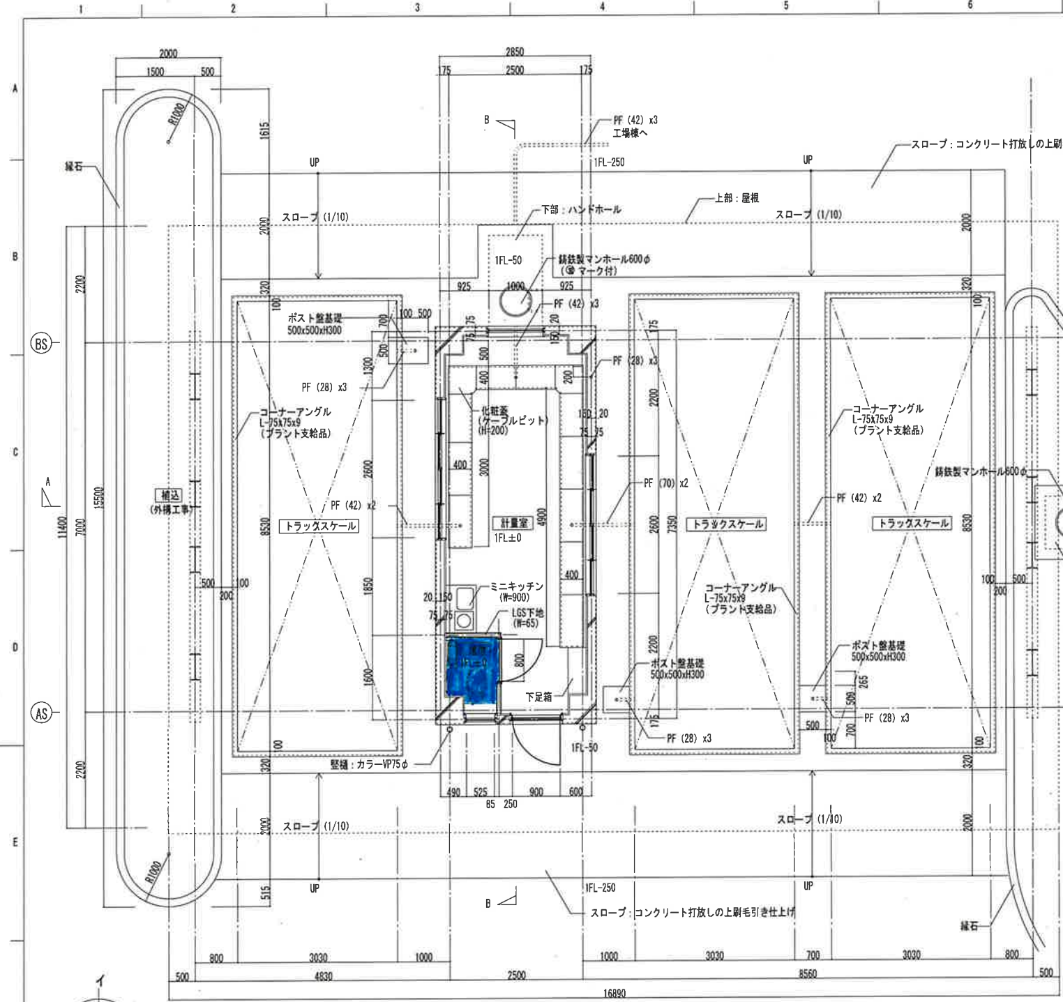
平面詳細図 1:50 (IFL-GL+250)
