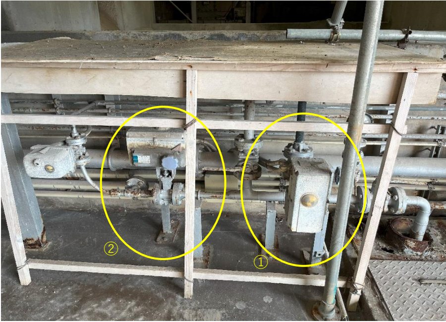
灰污水移送・戻り弁既設状況
