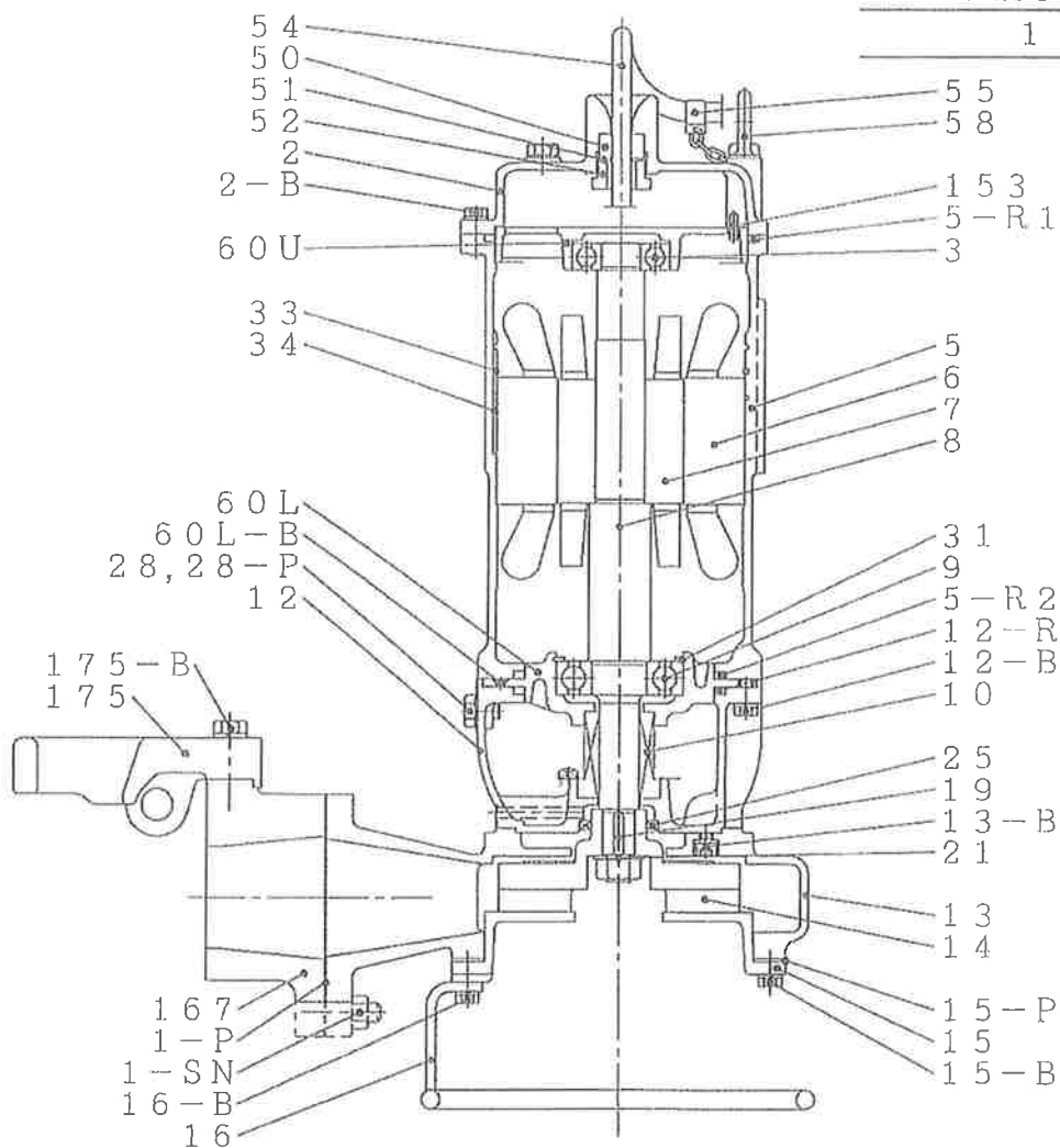
構造図部品表
